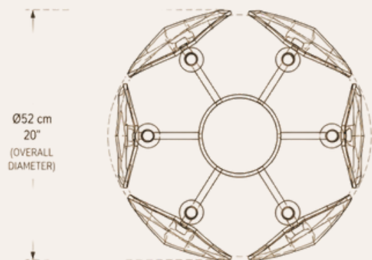
TOP ELEVATION
